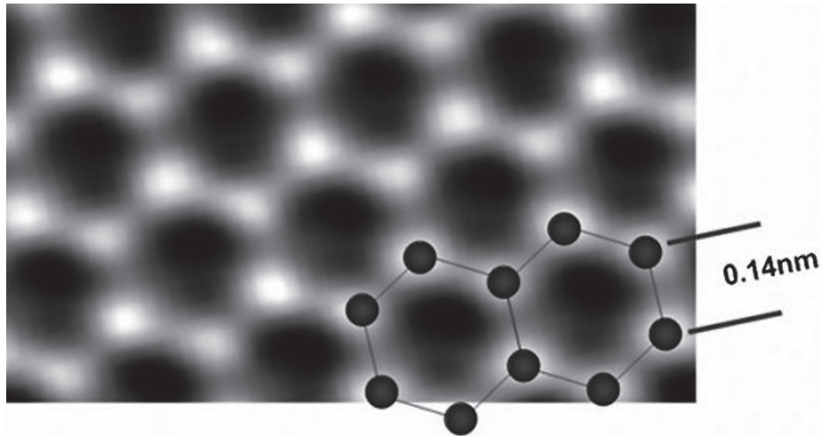
A képen a grafit kristályrácsának egy részlete látszik. A szénatomok homályos pontok. Ma ezt látjuk az atomi világból
